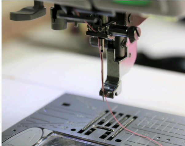
Setze den Knopflochfuß ein.
